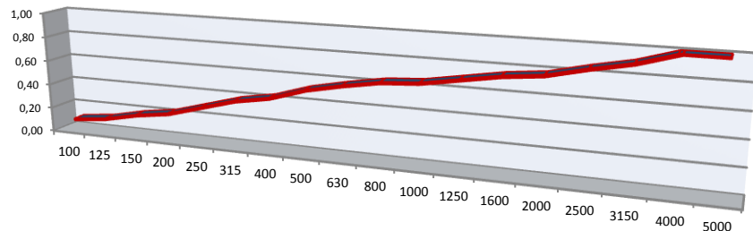
Diagrama 1: Absorção sonora em função da espessura, de acordo com a norma (Camara reverberante).
